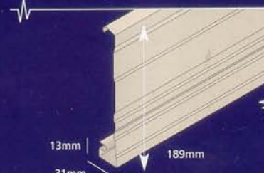
Stramit® Metal Fascia
